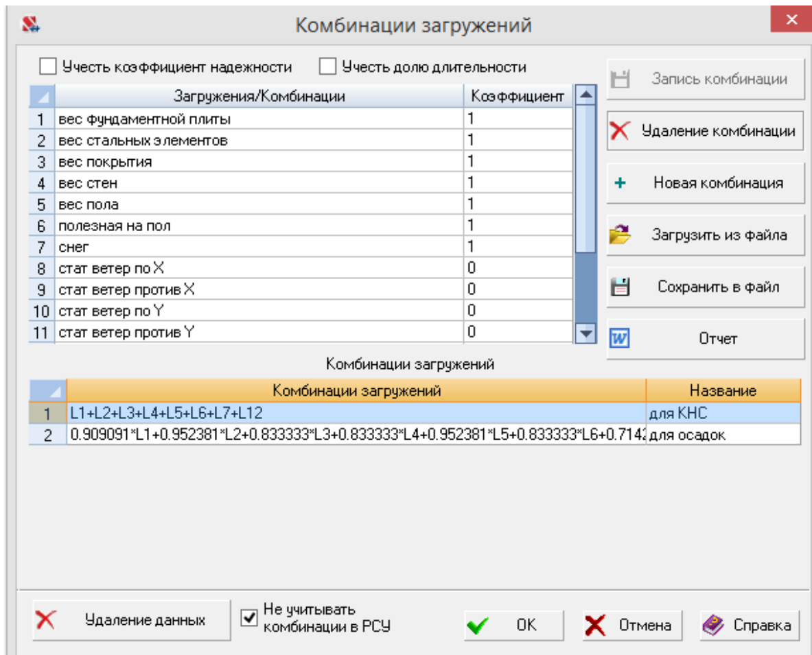
Рис. 3.6. Комбинация нормативных нагрузок для анализа деформаций
