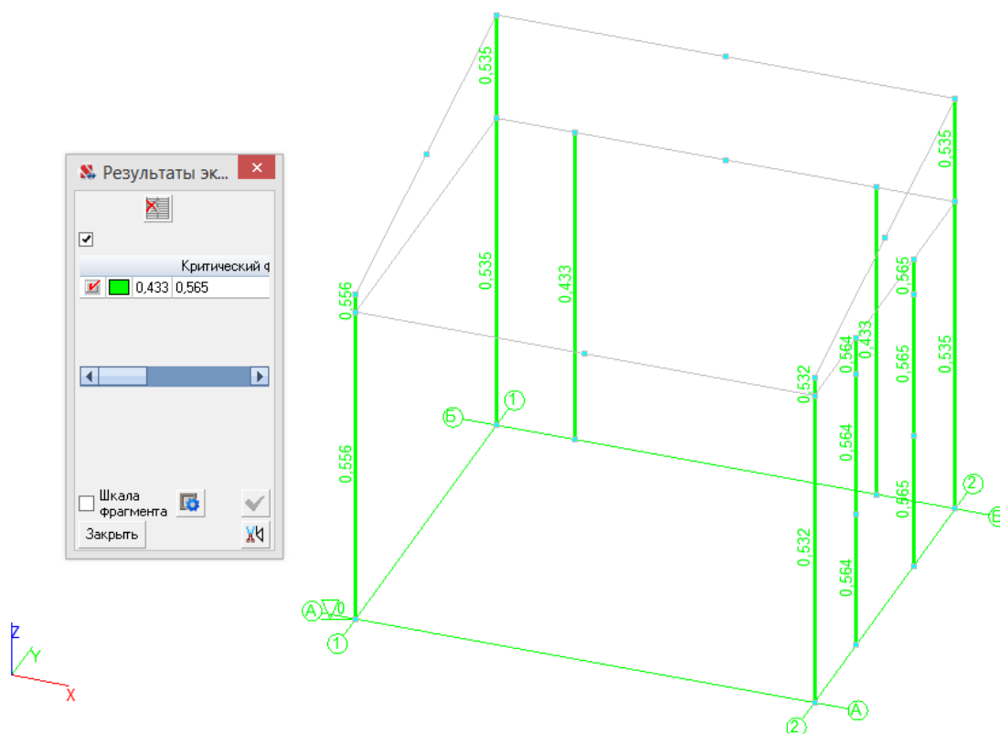
Рис. 3.7. Критический фактор K_{max} для колонн
