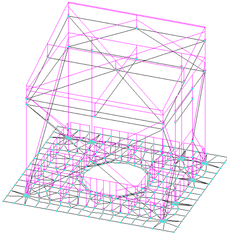
Рис. 3.3. Общий вид загрузки от веса элементов расчетной схемы (стального каркаса)
